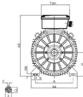
IM B3
