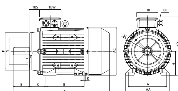
IM B34
