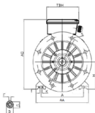
IM B3/B5
